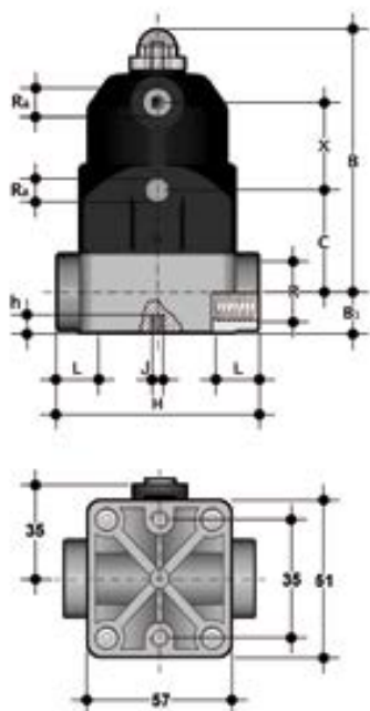
Компактный мембранный клапан CM с пневмоприводом НО с резьбовыми окончаниями (уплотнение FKM/мембрана PTFE) PP-H R1/2" (DN15)
