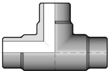
Тройник равнопроходной для стыковой сварки PP-H FIP (PN6) d110 SDR17.6 PN6
