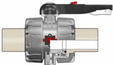
Шаровой кран VKD ПВДФ с длинными патрубками, DN65-110 d90 (DN80)
