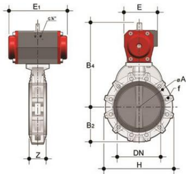
Дисковый затвор промышленного применения FK ПВХ с пневмоприводом ДвД, FKM, FIP d12" (DN300)
