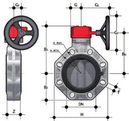
Дисковый затвор ПВХ FKOVRM с редуктором, FKM, FIP d75 (DN65)
