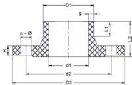
Фланцевое соединение жесткое для стыковой сварки PP-H IPS d355 PN10
