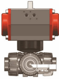
3-х ходовой шаровой кран ТКД ПВХ с пневмоприводом, Т-шар, FIP d50 (DN40)
