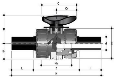
Шаровой кран для регулирования потока VKR с партрубками из ПЭ (уплотнение FKM) PP-H d40 (DN32)
