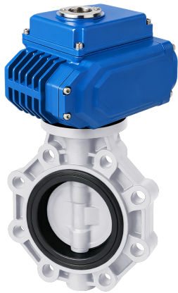
Дисковый затвор IFK ПВДФ с электрическим приводом 220V AC, FKM, IPS d140 (DN125)
