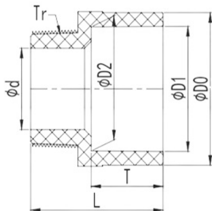
Муфта переходная с НР ПВХ IPS 63x2"
