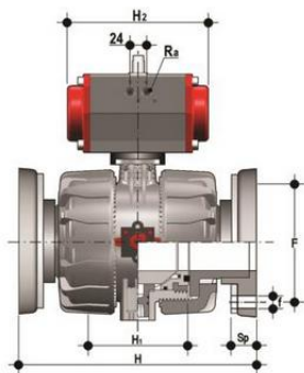
Шаровой кран VKD ПВДФ с пневмоприводом НЗ с фланцевыми окончаниями d110 (DN90)
