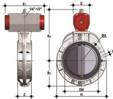
Дисковый затвор FK с пневмоприводом ДвД (уплотнение FKM) PP-H d14" (DN350)
