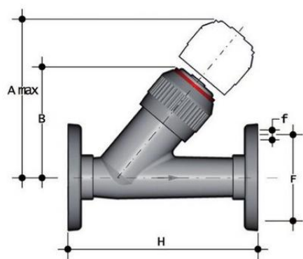
Угловой обратный клапан VROV PBX с фланцевыми окончаниями, EPDM, FIP d110 (DN100)
