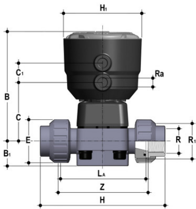
Мембранный клапан ДК ПВХ с пневмоприводом НЗ, PN6, резьбовые окончания, EPDM, FIP R3/4" (DN20)
