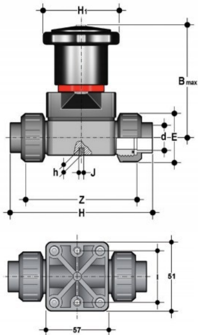
Компактный мембранный клапан ПБХ с пневмоприводом, CM, FKM, FIP R3/8" (DN12)
