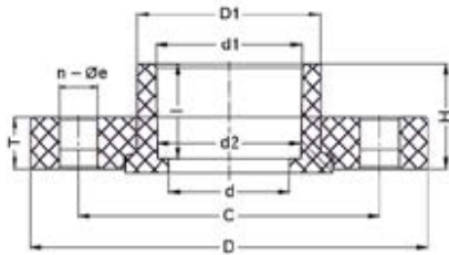
Фланец свободный с буртом ХПВХ IPS (Model A) d25 PN16
