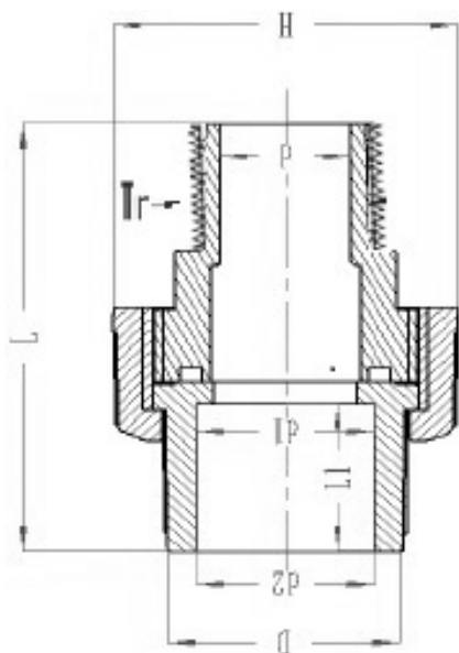
Муфта разборная с НР ПВХ IPS 25x3/4"
