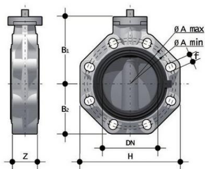
Дисковый затвор промышленного применения FKOAMFM со свободным штоком (уплотнение FKM) PP-H d16" (DN400)
