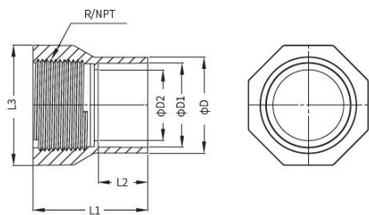
Редукционная муфта ПВДФ с ВР для стыковой сварки 20х1/2" PN 16
