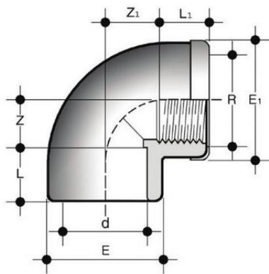
Отвод 90° переходной на ВР ПВХ FIP 16x3/8
