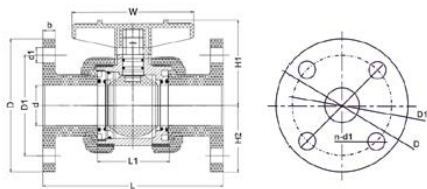
Кран шаровый ХПВХ фланцевые окончания промышленный EPDM IPS d40 (DN32)
