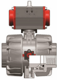
Шаровый кран промышленного применения VKD PBX с пневмоприводом, EPDM, FIP R2 1/2" (DN65)
