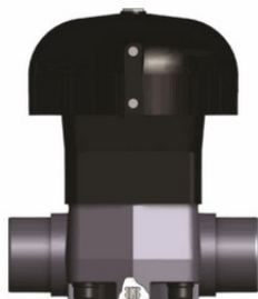
Мембранный клапан VM с пневмоприводом НО с втулочными окончаниями (уплотнение FKM/мембрана FKM) PP-H d90 (DN80)
