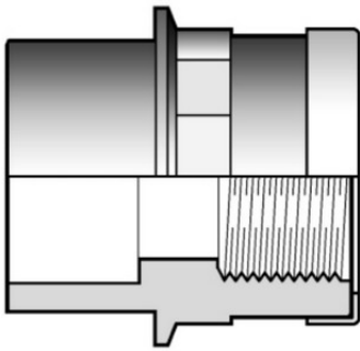
Двойной муфтовый адаптер с ВР и усиливающим кольцом ПВХ FIP 63x50x1 1/2
