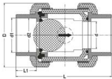
Обратный клапан ХПВХ шаровой IPS d32 (DN25)
