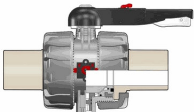
Шаровой кран VKD ПВДФ с длинными патрубками, DN65-110 d75 (DN65)
