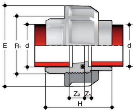
Муфта разборная ПВХД d32 SDR21 PN16
