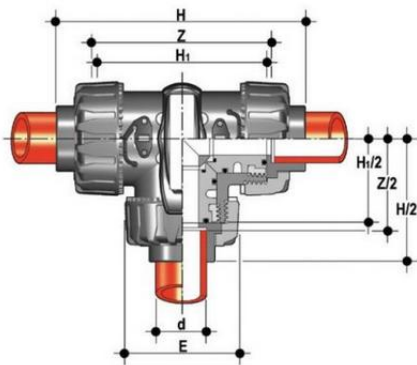
3-х ходовой шаровой кран ТКД с муфтовыми окончаниями Т-шар (уплотнение EPDM) PP-H d50
