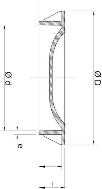
Фланцевая заглушка PPs d225
