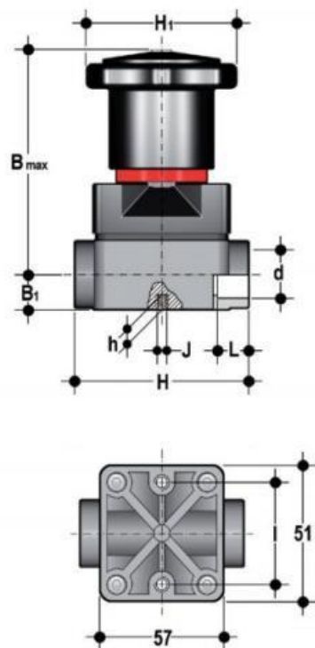
Компактный мембранный клапан ПВХ с пневмоприводом, CM, FKM, FIP d16 (DN10)
