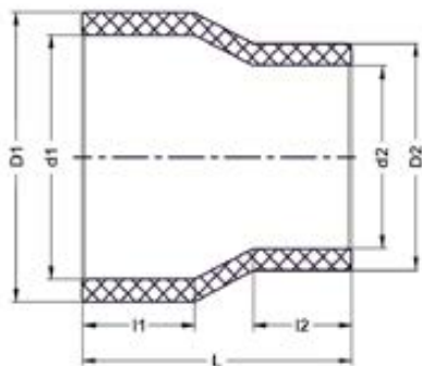
Муфта переходная для стыковой сварки PP-H IPS (Model B) 160x140 PN10
