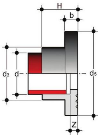
Бурт для раструбной сварки PP-H FIP d25 PN10
