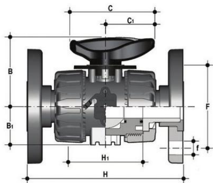
Шаровой кран для регулирования потока VKR с фланцевыми окончаниями (уплотнение FKM) PP-H d50
