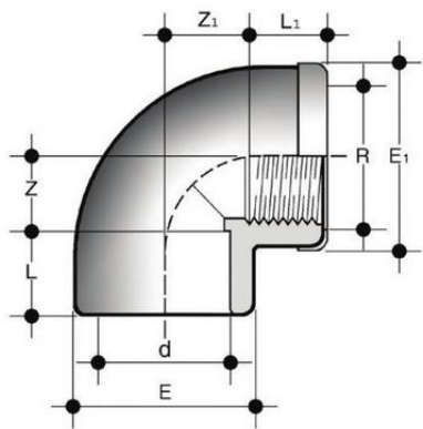
Отвод 90° переходной на ВР с кольцом ПВХ FIP 20x1/2
