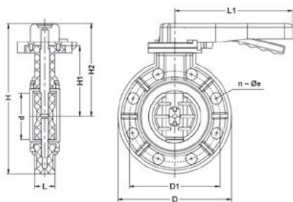
Затвор дисковый ПВХ с рукояткой общего применения EPDM IPS 110 (DN100)
