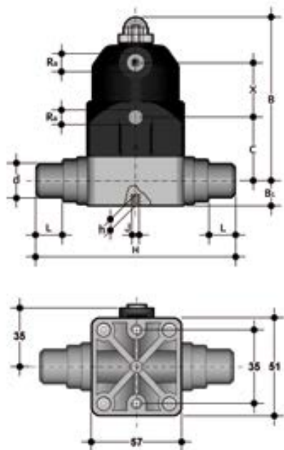
Компактный мембранный клапан СМ ПВДФ с втулочными окончаниями d20 (DN15)
