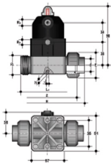
Компактный мембранный клапан PBX с пневмоприводом, CM, FKM, FIP d20 (DN15)
