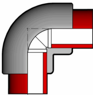
Отвод 90° для раструбной сварки PP-H FIP d63 PN10
