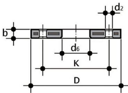
Свободный фланец PP-H FIP (PN16) d25 PN16
