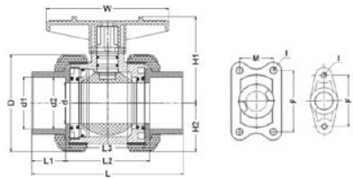
Кран шаровый ХПВХ муфтовый промышленный EPDM IPS d40 (DN32)
