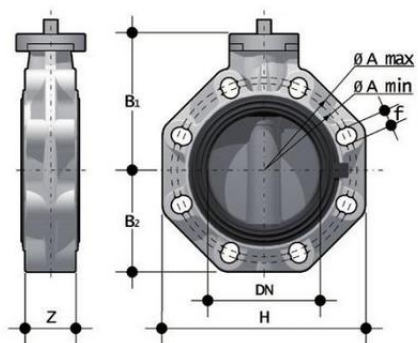
Дисковый затвор ПВХ FKOVFM со свободным штоком, EPDM, FIP d400 (DN400)
