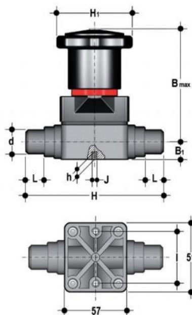
Компактный мембранный клапан CMDV PBX с втулочными окончаниями, FKM, FIP d20 (DN15)
