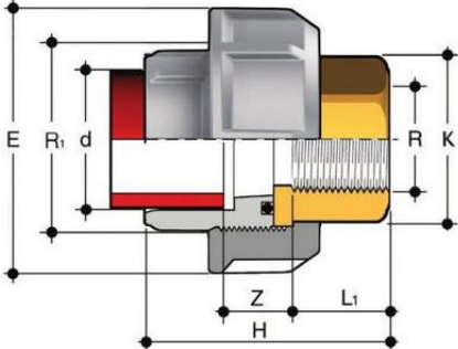
Муфта разборная переходная PP-H / латунь, ВР (EPDM) FIP 63x2 PN10
