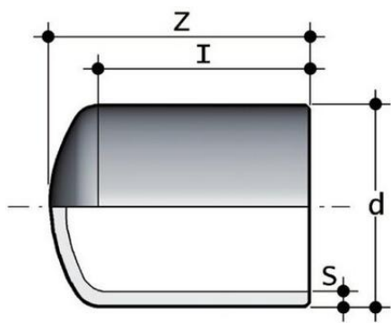
Заглушка для стыковой сварки PP-H FIP (PN6) d225 SDR17.6 PN6
