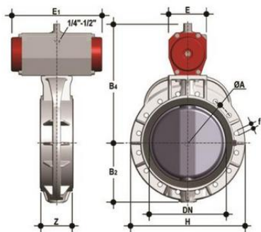
Дисковый затвор FK с пневмоприводом ДвД (уплотнение FKM) PP-H d355 (DN350)
