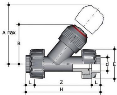
Угловой обратный клапан VRUIV PBX с разборными муфтовыми окончаниями, EPDM, FIP d25 (DN20)
