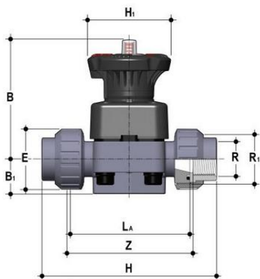
Мембранный клапан ДК ХПВХ с разборными резьбовыми окончаниями R1" (DN25)
