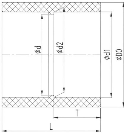
Муфта соединительная ПВХ IPS d32
