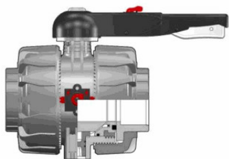
Шаровой кран промышленного применения VKD ХПВХ с муфтовыми окончаниями, DN65-100 d90 (DN80)
