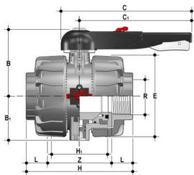
Шаровый кран промышленного применения VKD ХПВХ с резьбовыми окончаниями, DN65-100 R4" (DN90)
